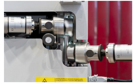
Automatic knife sharpening Afilado automatico de cuchilla
