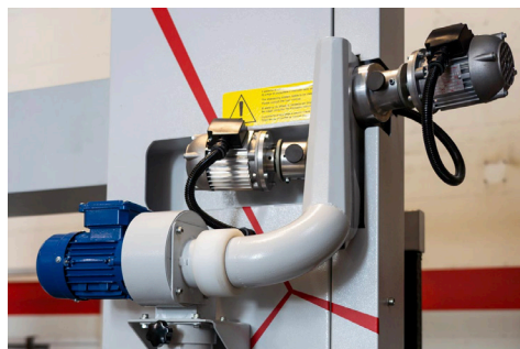
Air blowing system for blade cleaning and cooling / Sistema de soplado para limpieza y refrigeración de cuchilla
