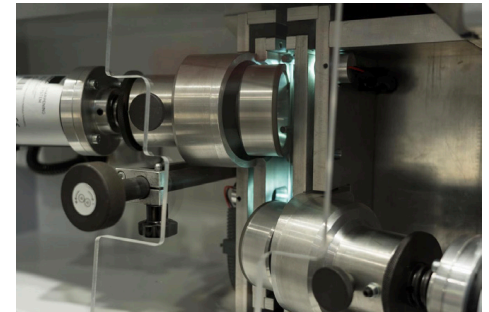
Automatic knife sharpening Afilado automatico de cuchilla
