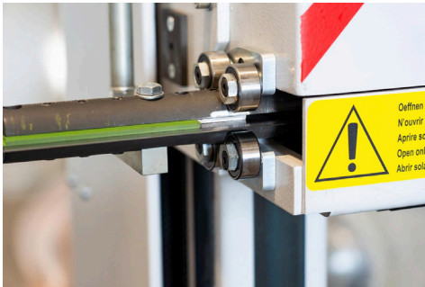
Automatic tilting blade guide / Guiado automático de cuchilla bas-culante
