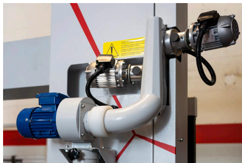
Air blowing system for blade cleaning and cooling / Sistema de soplado de aire para la limpieza y refrigeración de la cuchilla
