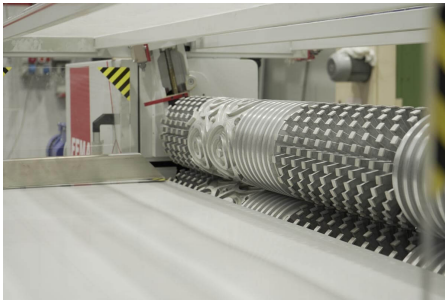
1385-7ZR Zones Patterns Roller set 1385-7ZR Juego de rodillos de siete zonas
