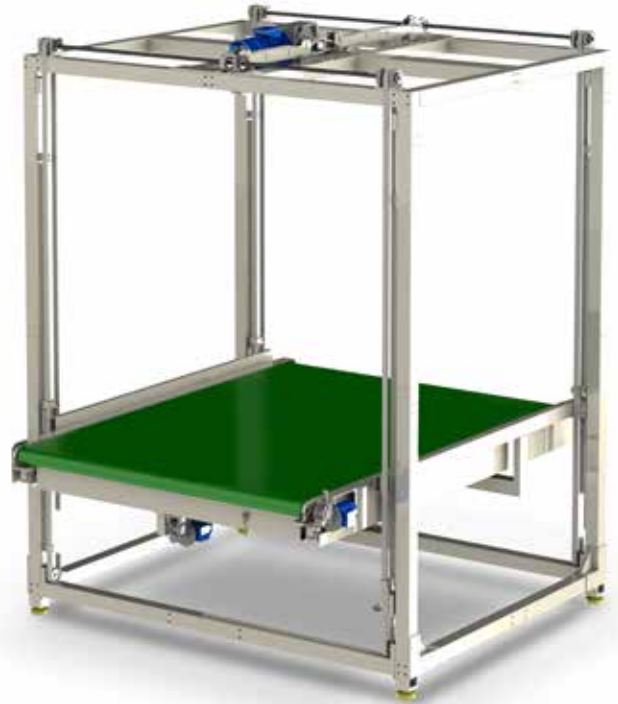
H290 DS - Mattress Destacker Desapilador de Colchones
