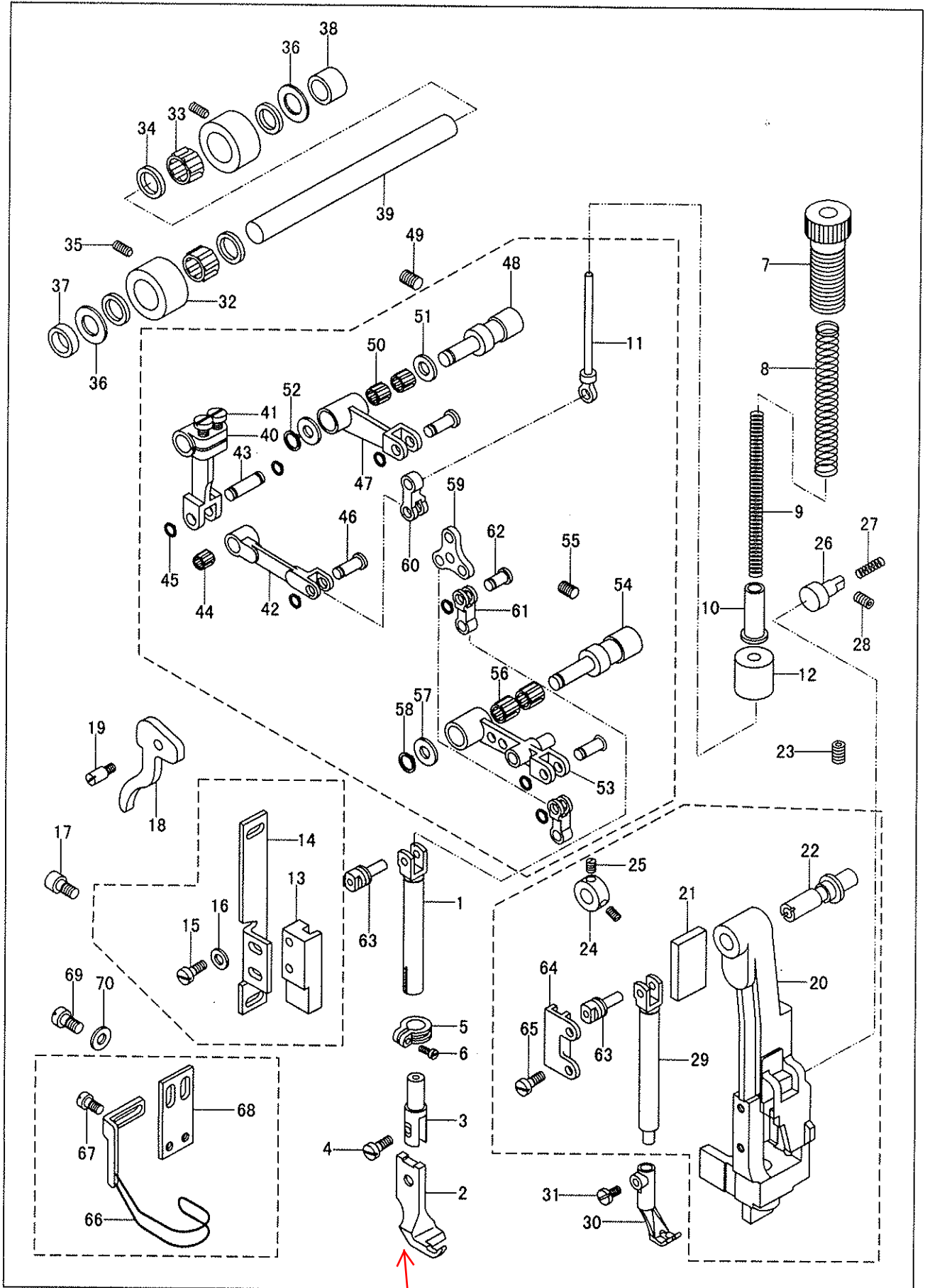
1245-46970 Fuß 2 Schenklig
