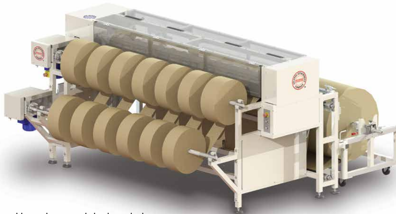
1393SBS Con cerrador de bolsa opcional y doble enrollador
